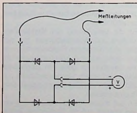
Bild 1: Bei jeder Polung Zeigerausschlag
