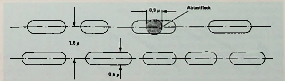
Bild 5: Informationsspur und Abtastfleck einer CD-Disc
