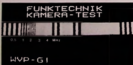
Bild 4: Horizontale Auflösung Kamera-Ausgang ( E > 1400 Lux)
