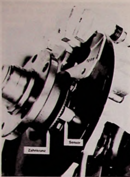
Bild 4: Sensor am Hinterrad als Signalgeber für das Eva-System (Blaupunkt-Pressbild)
