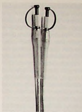
Bild 1: Lichtwellenleiter-Kabel mit geschützten Steckverbindungen (Reinshagen-Pressbild)
