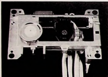
Bild 2a: CD-Laufwerk mit optischem Abtaster, Antriebssystem für radiale Regelung und Disc-Motor (Thomson-Brandt-Pressbild)
