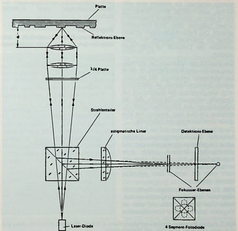
Bild 4: Schematischer Strahlengang eines optischen Abtasters
