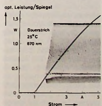
Bild 1: Laserdioden-Array mit hoher optischer Ausgangsleistung (Siemens-Pressbild)
