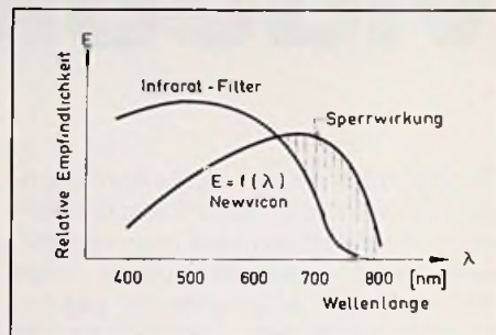
Bild 6: Die Wirkung des in den Strahlengang eingefügten IR-Filters
